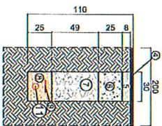
SEZIONE DI SCAVO
